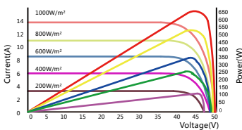
FS182*182-M-72-MH-530W
